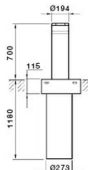
Reflektierende Folie H: 50 mm und Stahlzylinder der Farbe Grau RAL 7022 mit LED-Leuchtkranz hoher Lichtausbeute.
