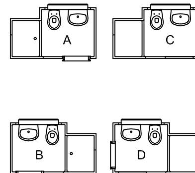
Type 17, Variante A-D Duschwanne mit Hochzug
